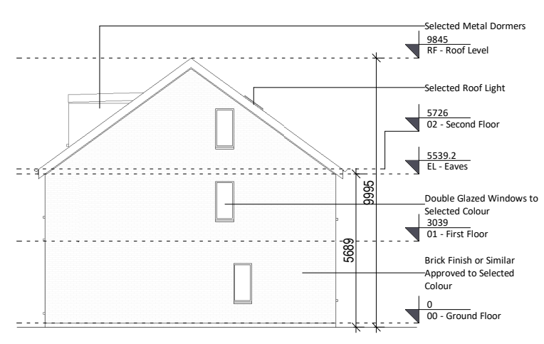
6 Right Elevation 1 : 200
