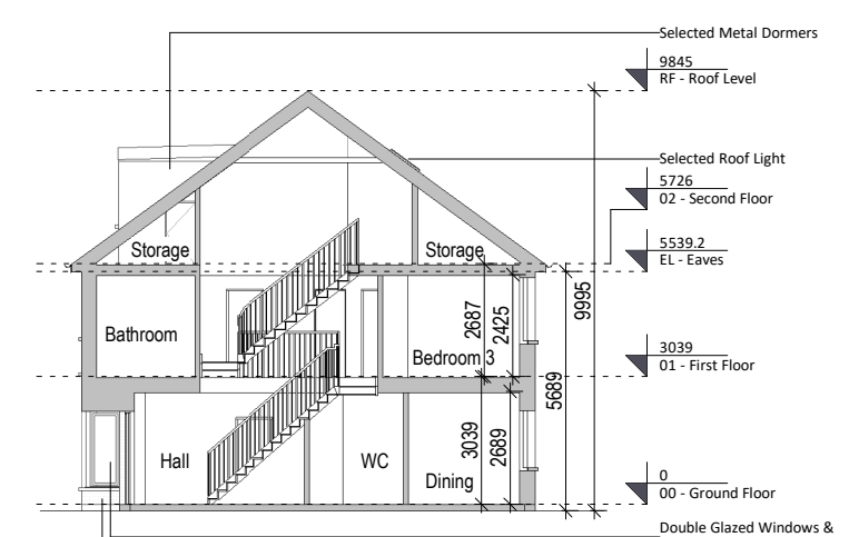
7 Section 1 1 : 200
